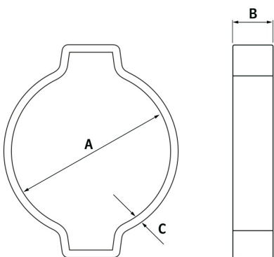
OETIKER 151 - OPASKI Z 2 USZAMI - W4
