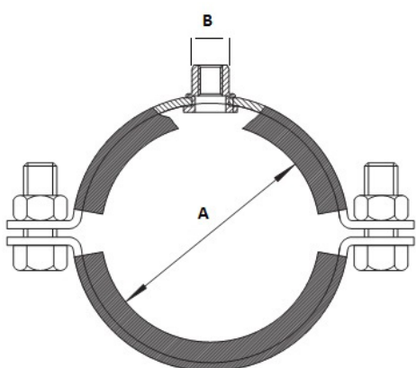
UCHWYTY DO RUR - HEAVY UNI M12/M16- W1 (do rur masywnych z okładziną EPDM)
